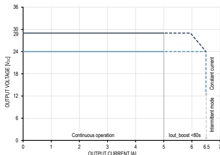
Fig. 4: Boost current capability up to 55°C amb
